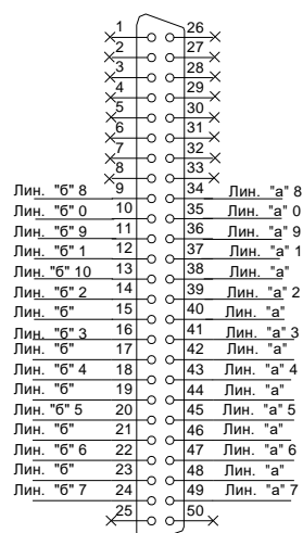
Модуль 16СТ, 8СТ (Лин. 0...7)
