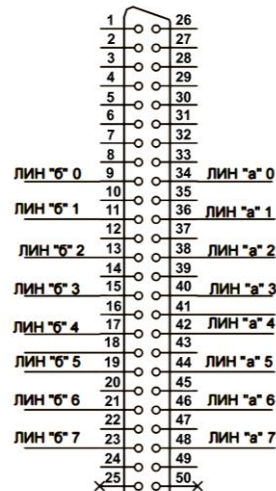
Модуль 8МБ
