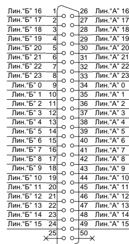
Модуль 24АК
