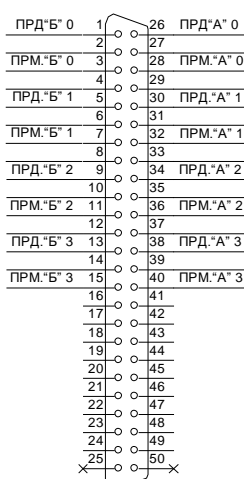
Разъем ХТ
