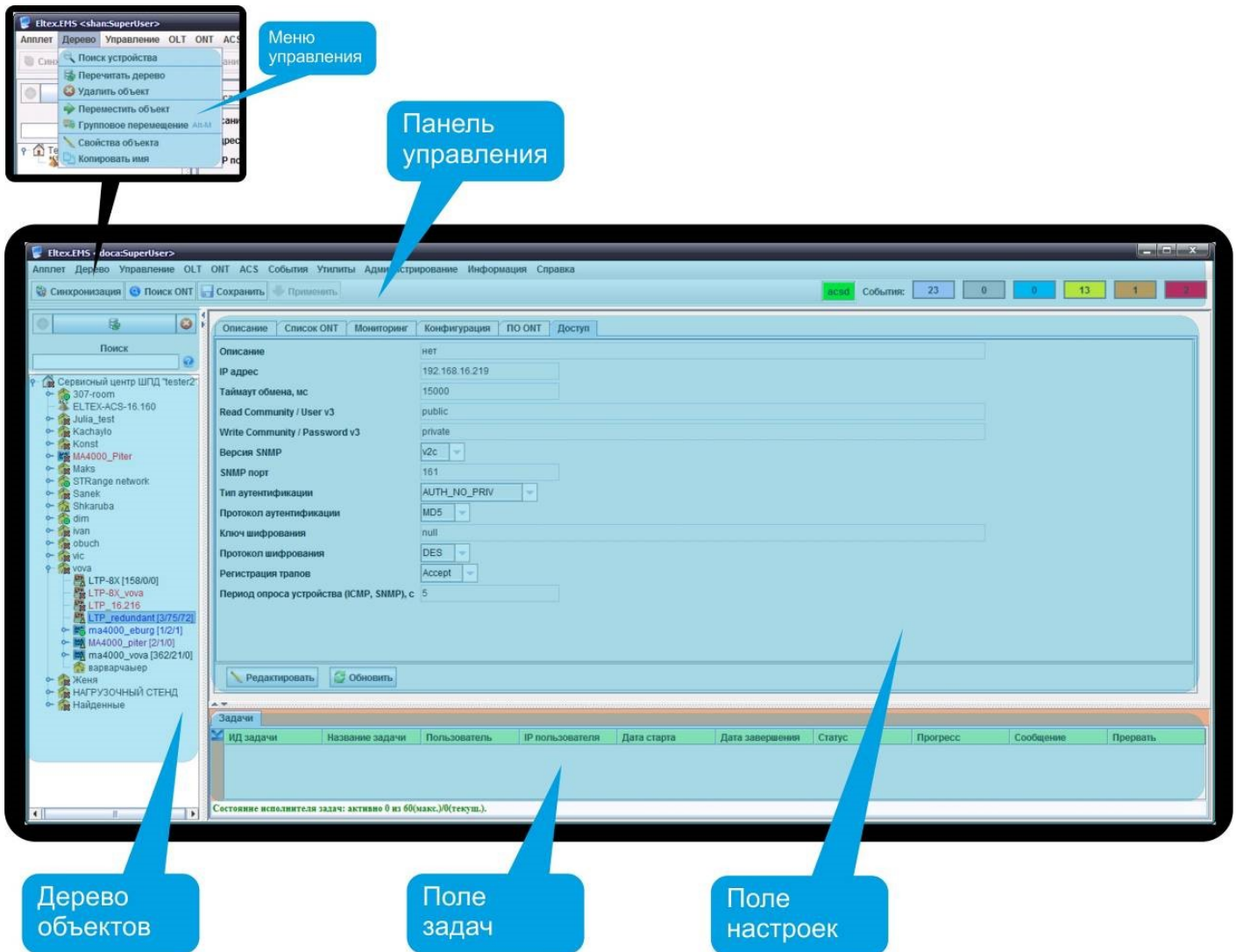
Рисунок 2 – Области навигации пользовательского интерфейса системы EMS.Eltex
