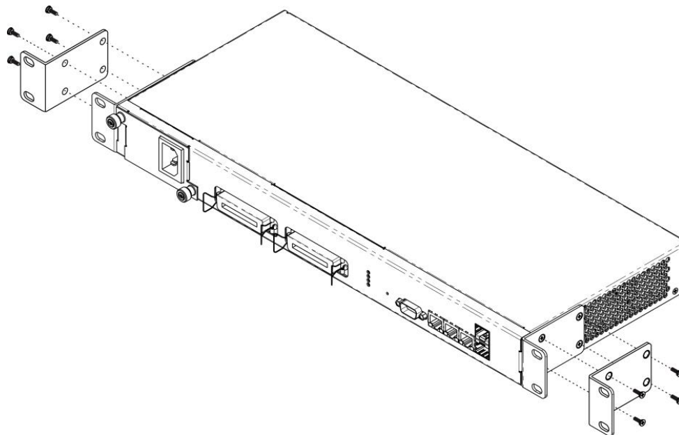
Рисунок 11 – Крепление кронштейнов
