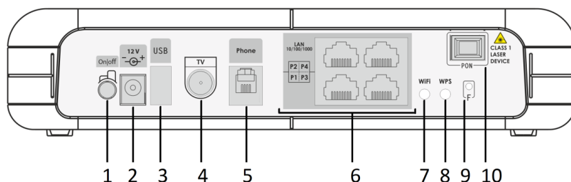
Рисунок 5 – Внешний вид задней панели NTU-RG-1421GC-Wac
