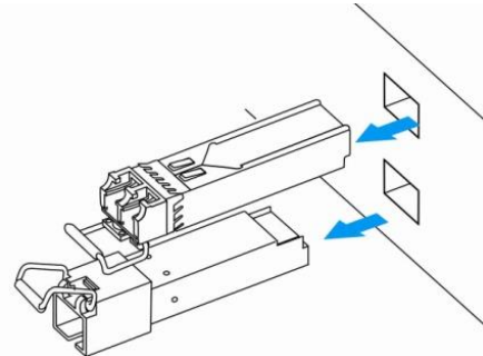
Рисунок 86 – Извлечение SFP-трансиверов
