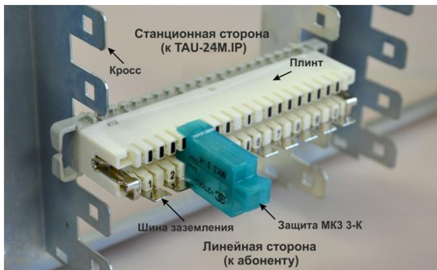
Рисунок 10 – Схема подключения
