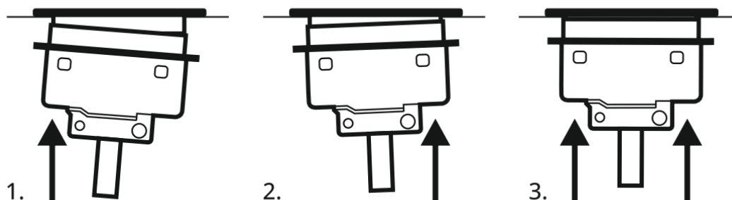
Рисунок 5 – Схема подключения разъема кабеля к ответной части на шлюзе
