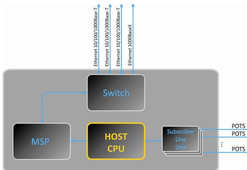
Рисунок 3 – Функциональная схема TAU-24/16.IP
