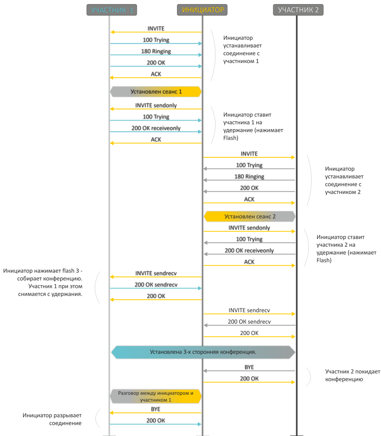
Рисунок 12 – Алгоритм выполнения услуги «Трёхсторонняя конференция» («3-way conference») локально на устройстве по протоколу SIP
