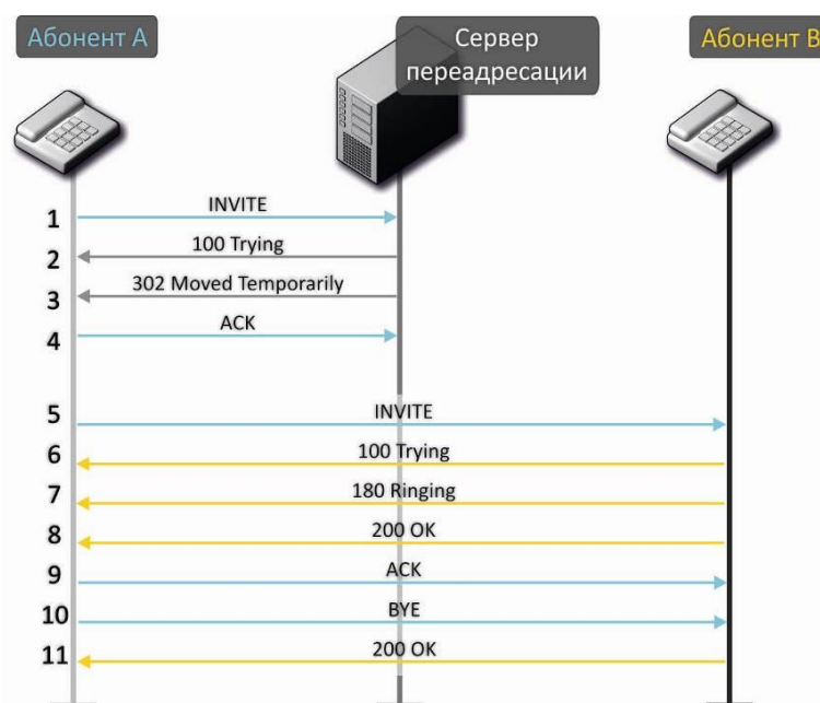
Рисунок 17 – Алгоритм вызова с участием сервера переадресации
