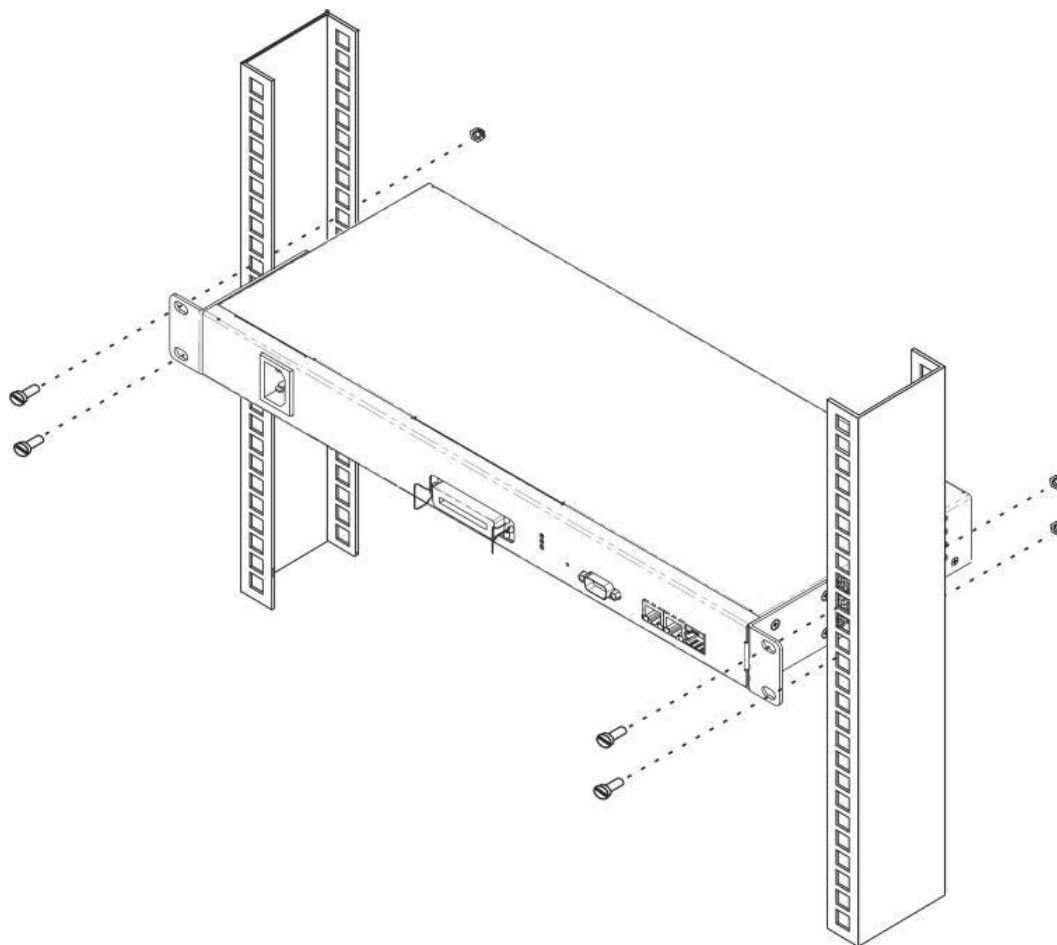
Рисунок 8 – Установка устройства в стойку
