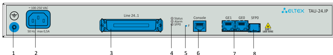
Рисунок 4а – Внешний вид передней панели TAU-24.IP с питанием от сети переменного тока
