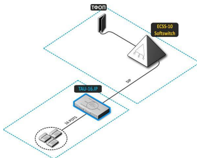
Рисунок 1 – Абонентский вынос на примере TAU-16.IP
