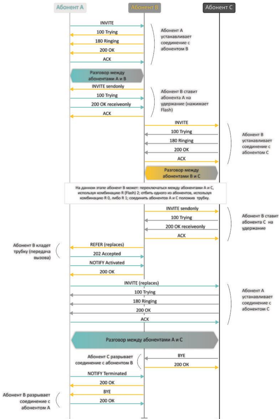
Рисунок 9 – Алгоритм выполнения услуги «Перевод вызова с сопровождением» (« Attended calltransfer ») абонентом В по протоколу SIP
