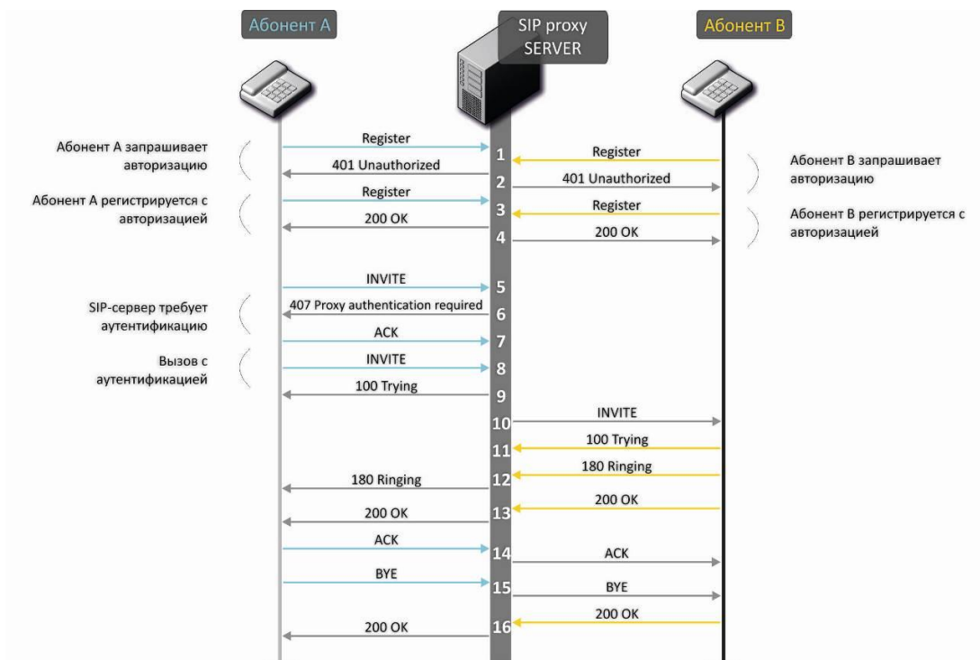
Рисунок 16 – Алгоритм вызова с участием SIP проху-сервера
