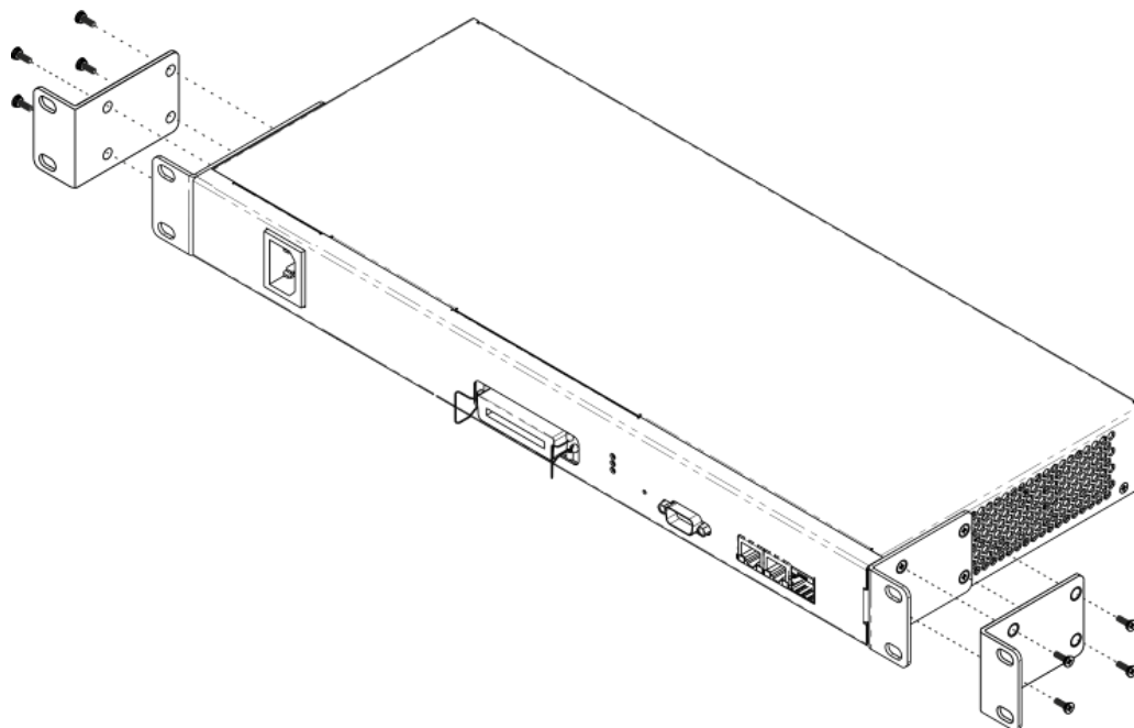
Рисунок 7 – Крепление кронштейнов
