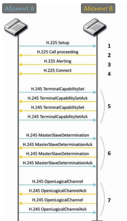
Рисунок 18 – Алгоритм вызова по протоколу H.323
