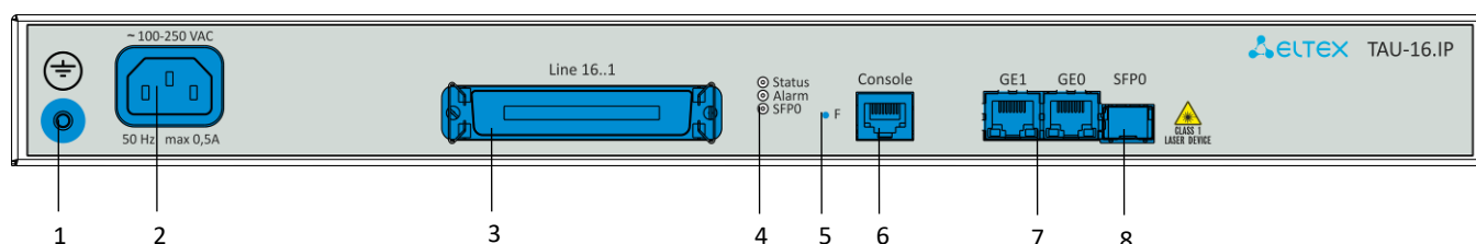
Рисунок 4б – Внешний вид передней панели TAU-16.IP с питанием от сети переменного тока
