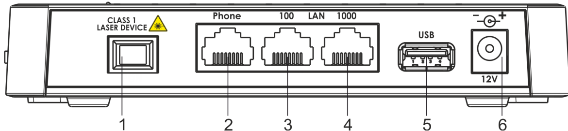
Рисунок 2 – Внешний вид задней панели NTU-52V
