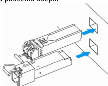
Рисунок 59 – Установка SFP-трансиверов
