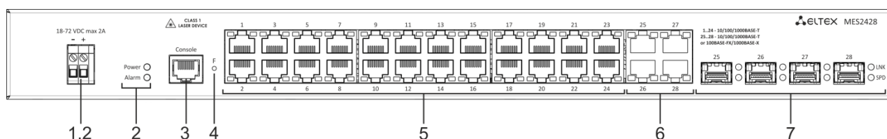
Рисунок 13 – Передняя панель MES2428 DC
