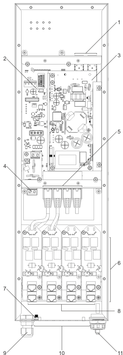
Рисунок 51 – Основные компоненты и разъемы MES3708P
