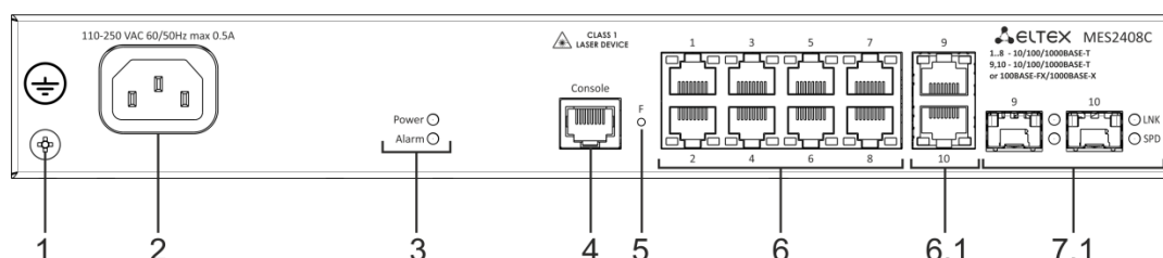
Рисунок 6 – Передняя панель MES2408C
