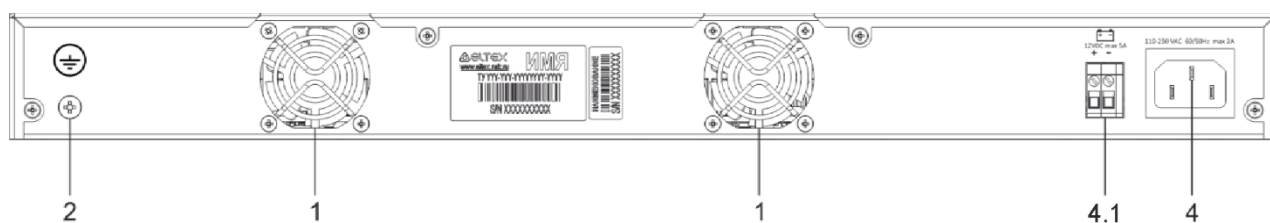
Рисунок 40 – Задняя панель MES2448B
