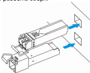
Рисунок 59 – Установка SFP-трансиверов
