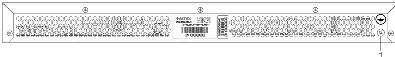
Рисунок 36 – Задняя панель MES1428, MES2428, MES2428B, MES2408IP DC1, MES2408P, MES2424 и MES2424B
