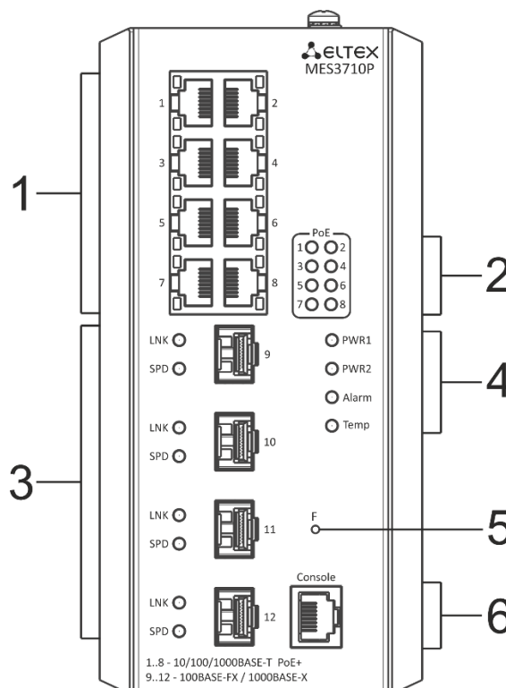
Рисунок 35 – Передняя панель MES3710P
