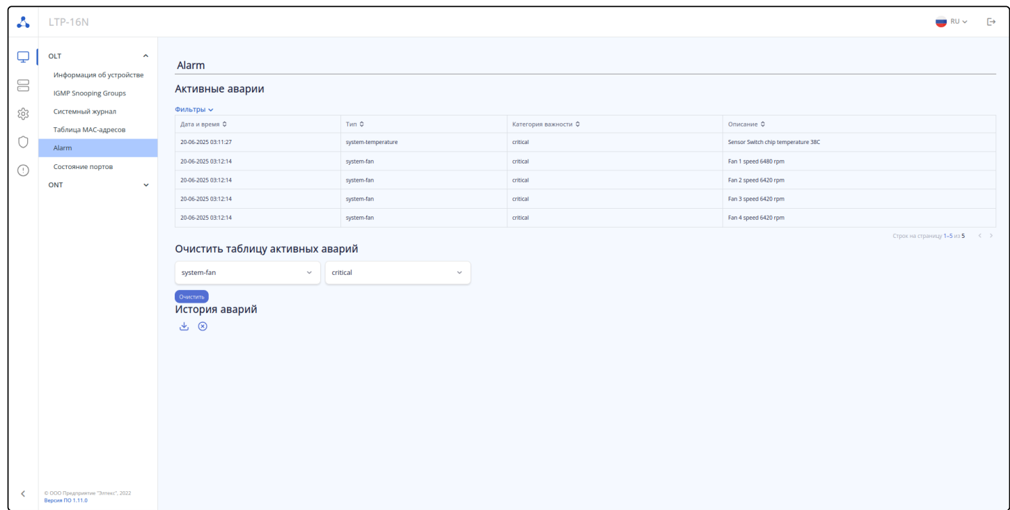
Рисунок 7 – Страница «Alarm»
