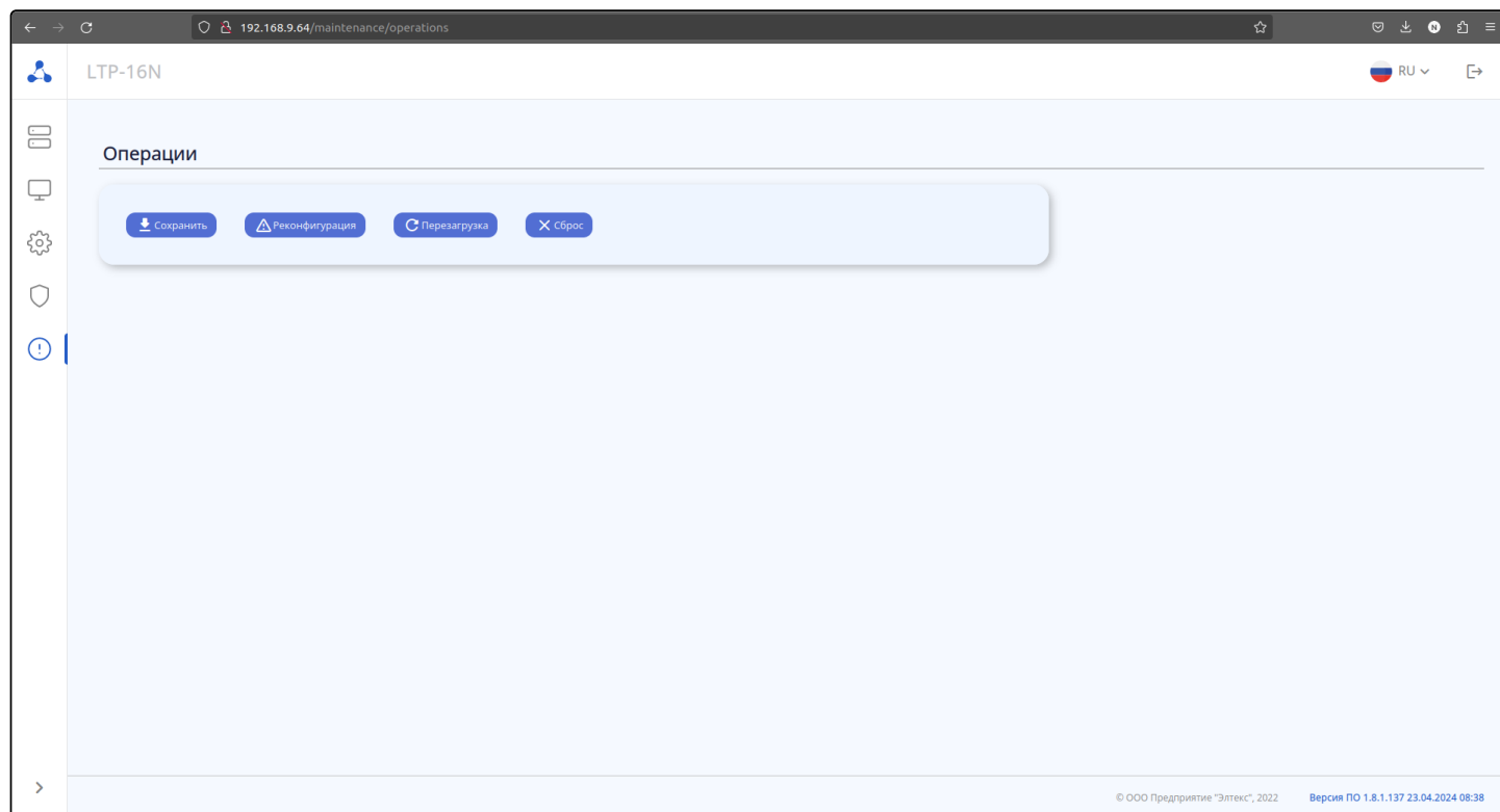
Рисунок 44 — Страница «Операции»
