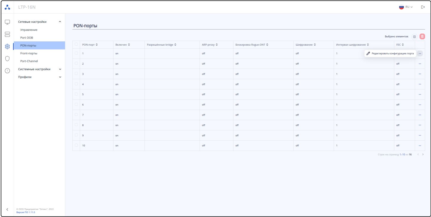
Рисунок 22 — Страница «PON-порты»
