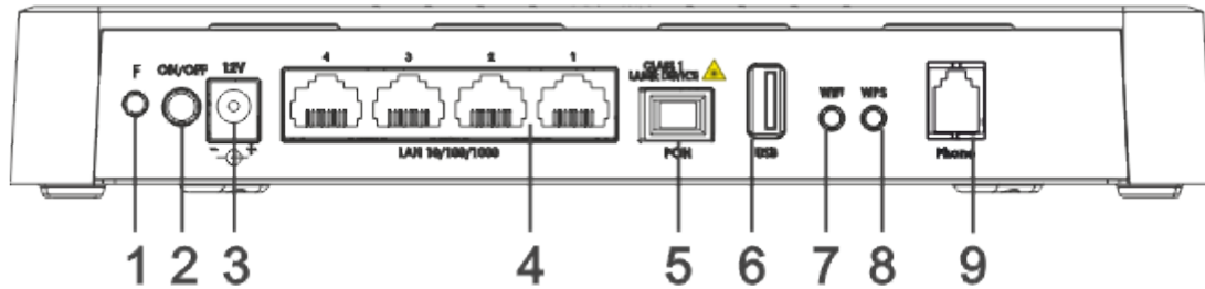
Рисунок 4 – Внешний вид задней панели NTU-RG-5521G-Wax, NTU-RG-5521G-Wax-Z
