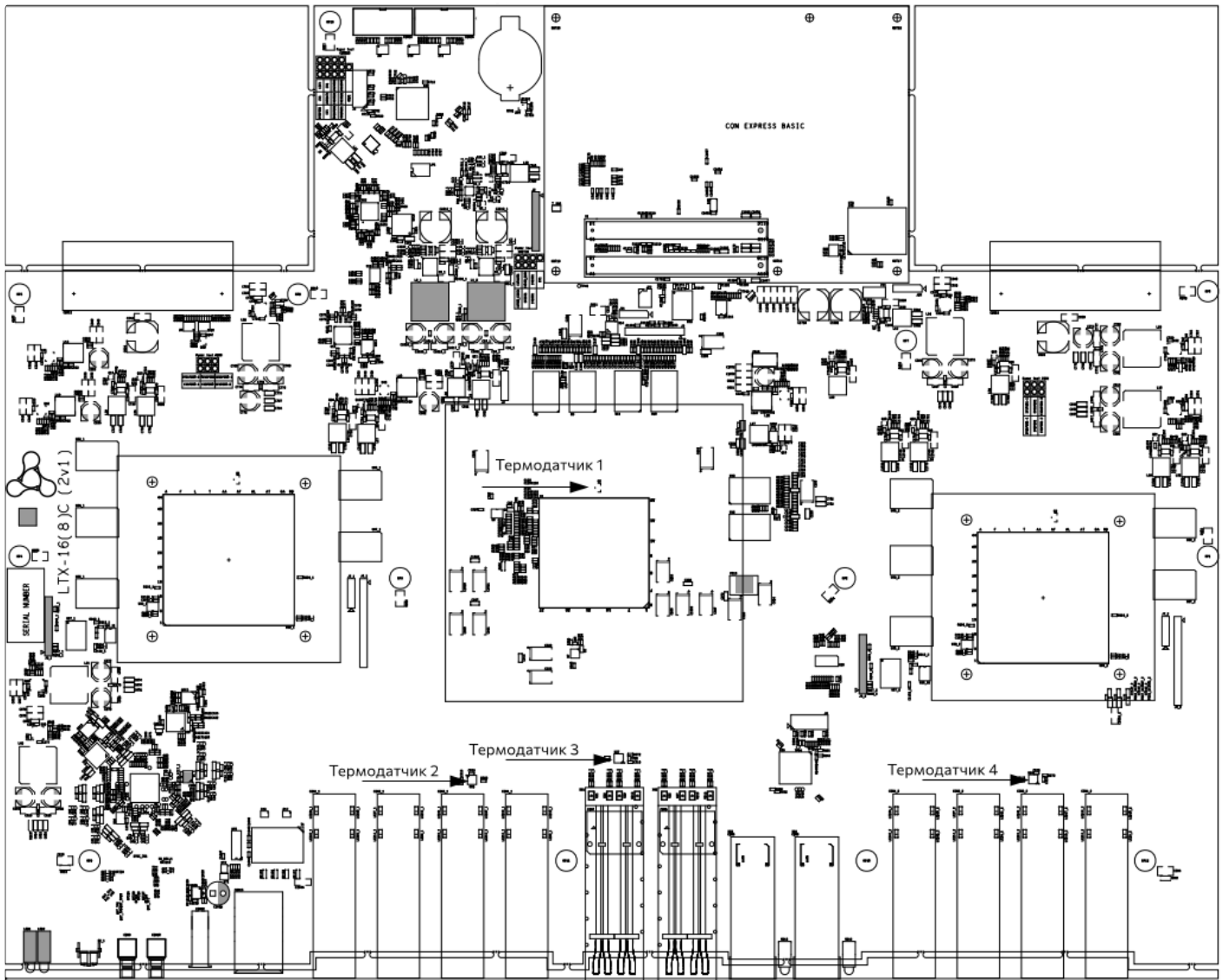
Рисунок 24 – Расположение термодатчиков LTX-8(16)C
