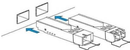
Рисунок 43 – Установка SFP-трансиверов
