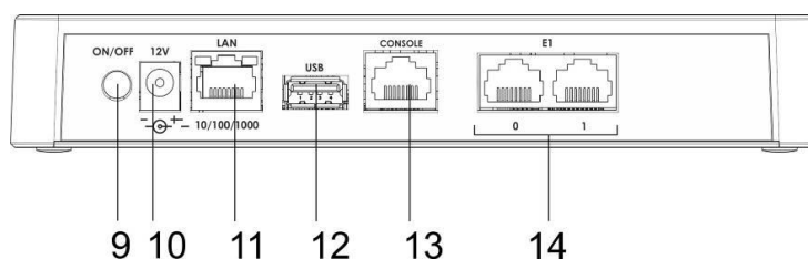
Рисунок 86 – Внешний вид SMG-2. Задняя панель
