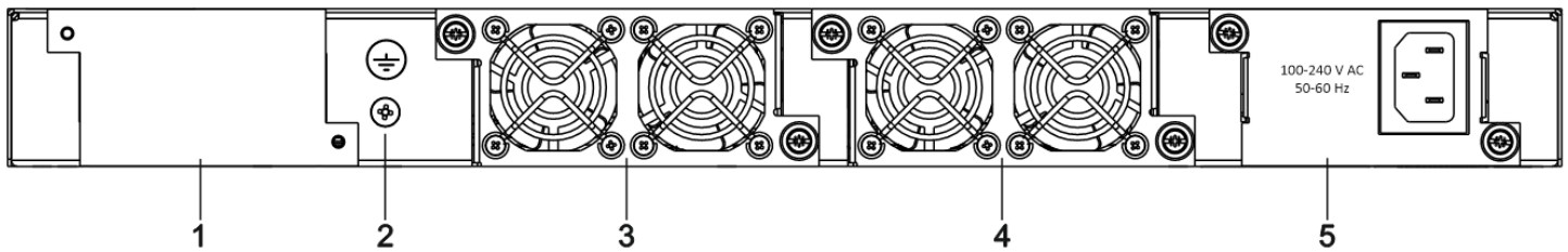
Рисунок 10 – Задняя панель ESR-3200
