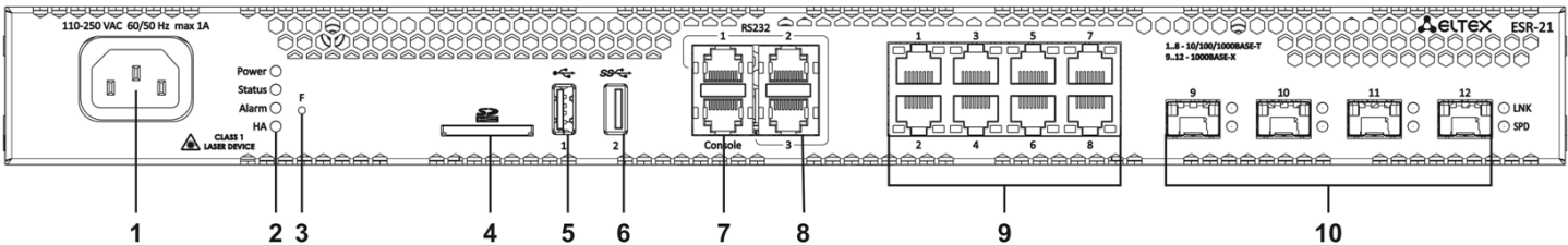
Рисунок 41 – Передняя панель ESR-21
