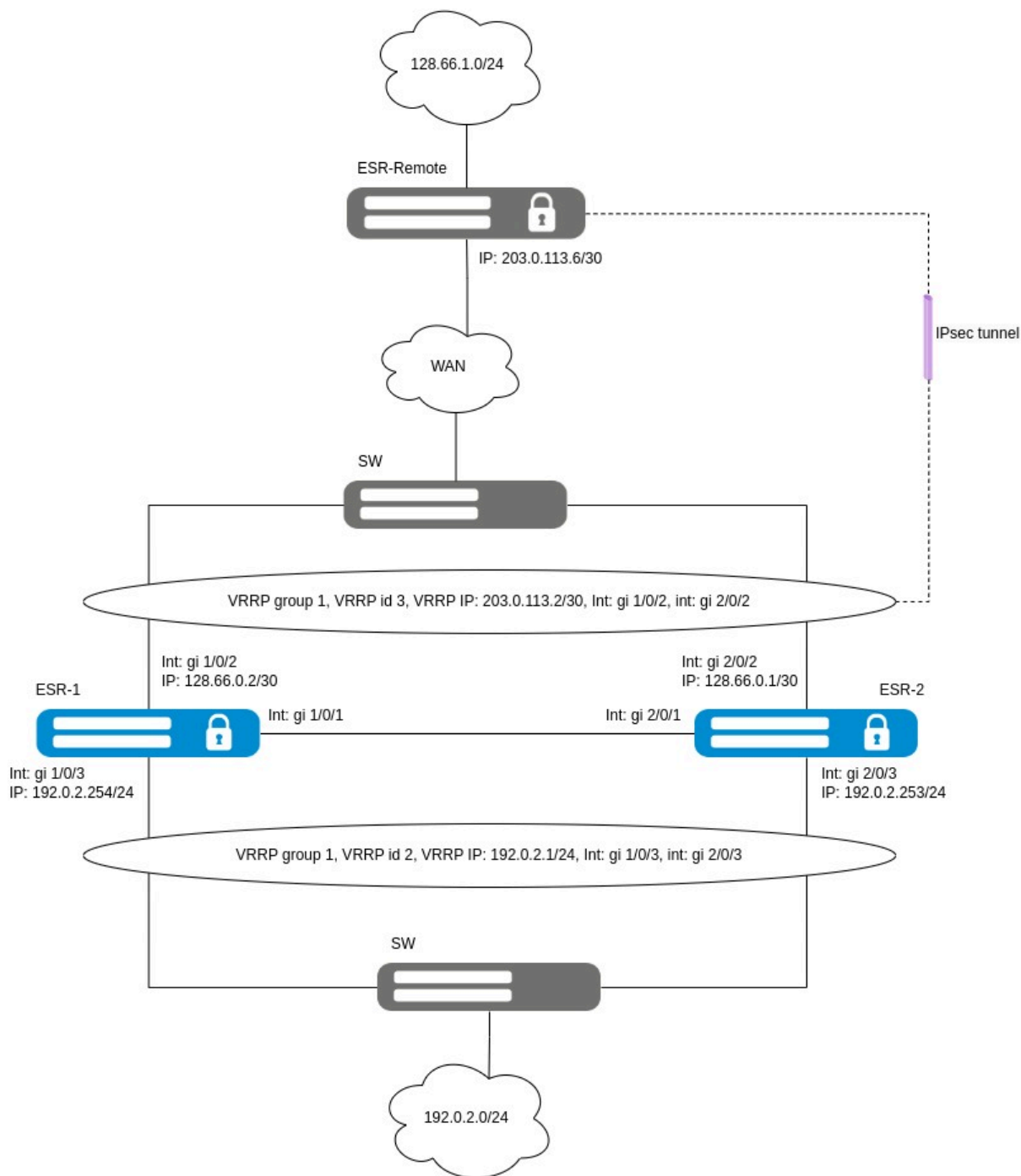
Схема реализации Route-based IPsec VPN
