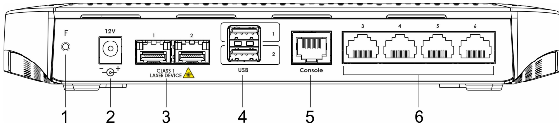
Рисунок 58 – Задняя панель ESR-15
