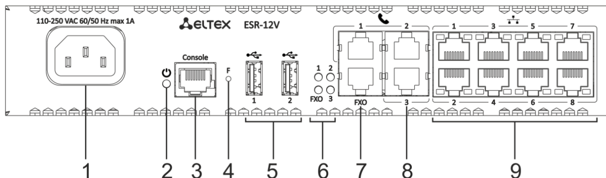
Рисунок 64 – Передняя панель ESR-12V
