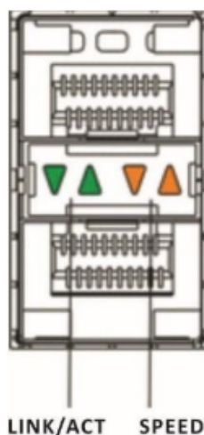
Рисунок 72 – Расположение индикаторов SFP/SFP+/SFP28-интерфейсов
