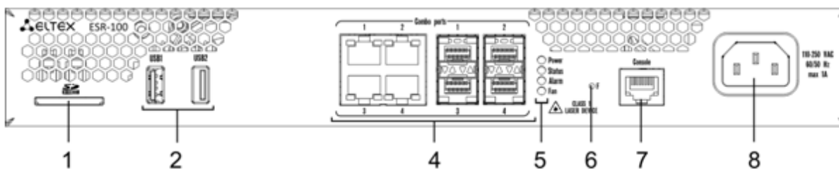
Рисунок 33 – Передняя панель ESR-100
