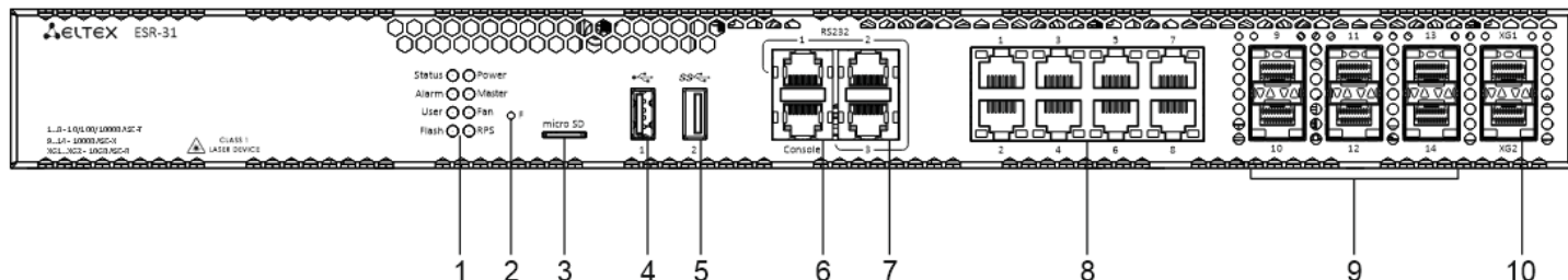
Рисунок 37 – Передняя панель ESR-31
