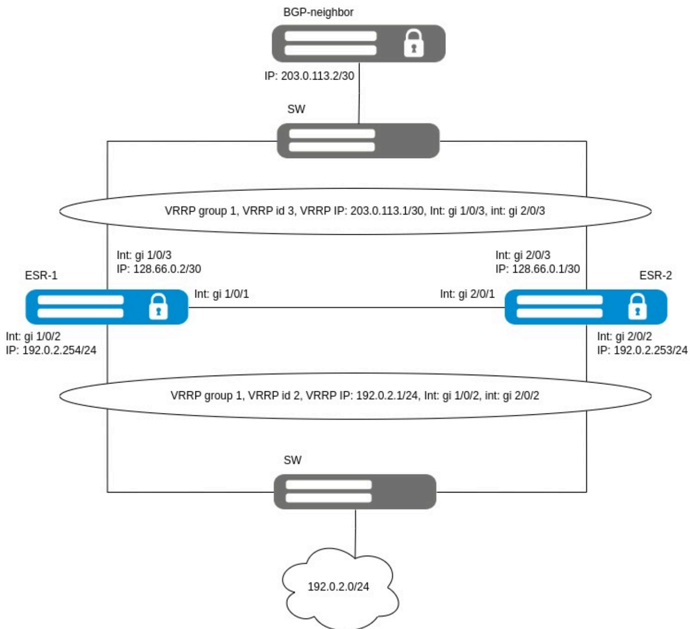
Схема реализации eBGP с общим IP-адресом
