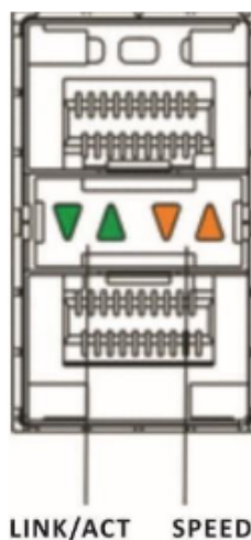
Рисунок 74 – Расположение индикаторов состояния SFP/SFP+/SFP28-интерфейсов
