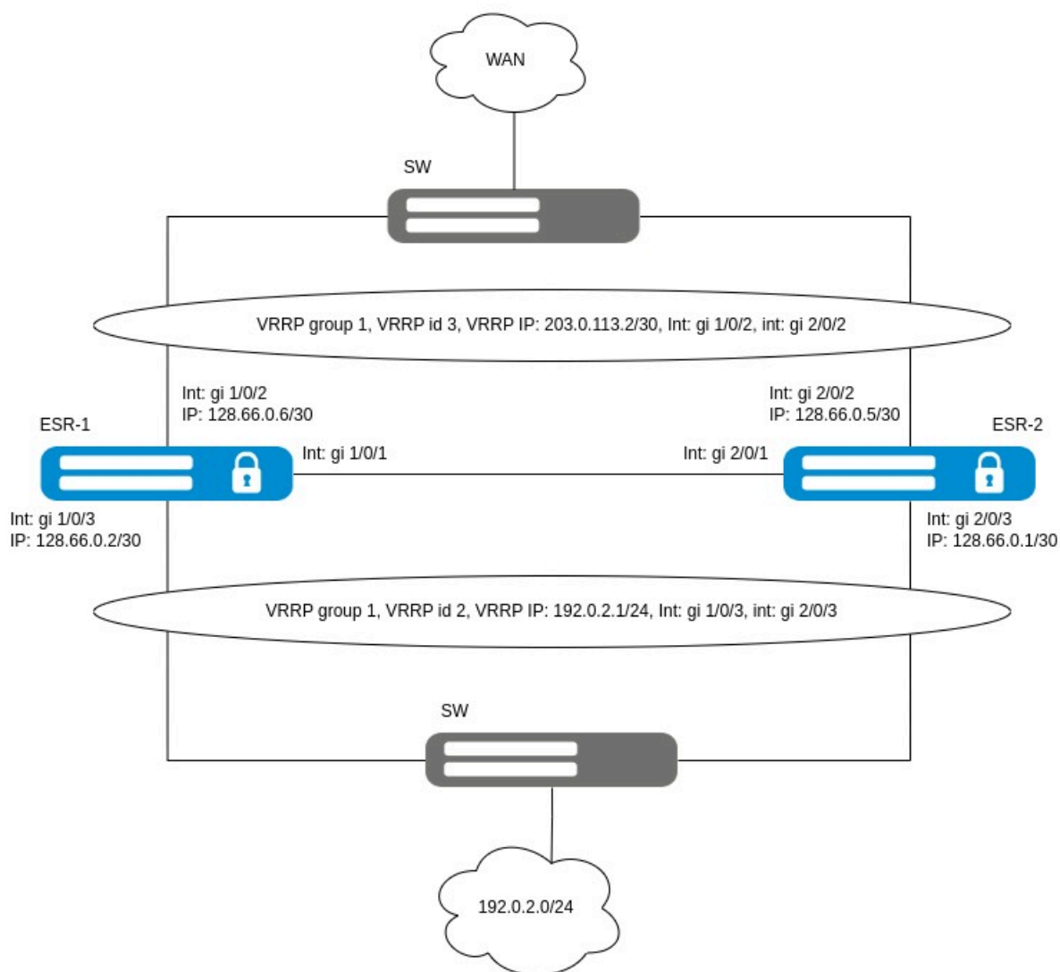
Схема реализации Destination NAT
