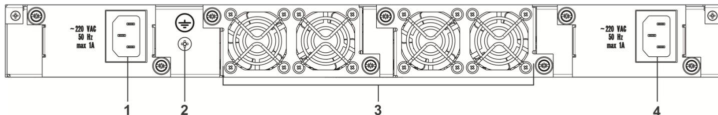
Рисунок 24 – Задняя панель ESR-1511 rev.B, ESR-1511, ESR-1500
