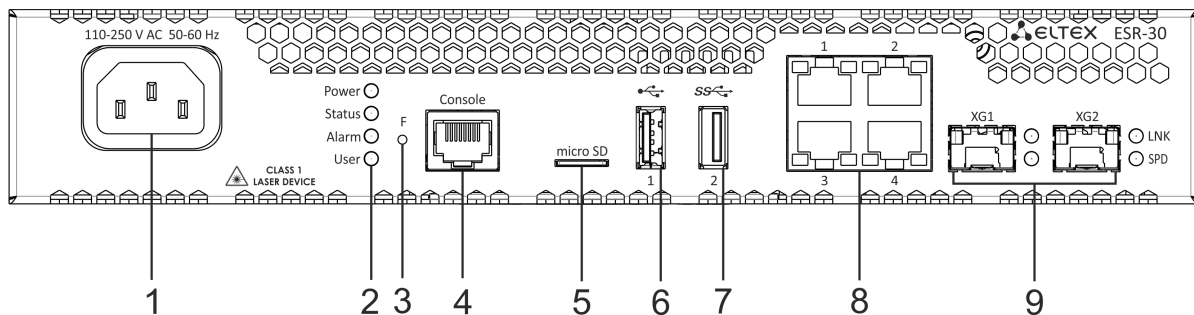
Рисунок 45 – Передняя панель ESR-30
