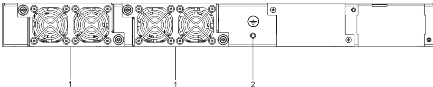
Рисунок 38 – Задняя панель ESR-31
