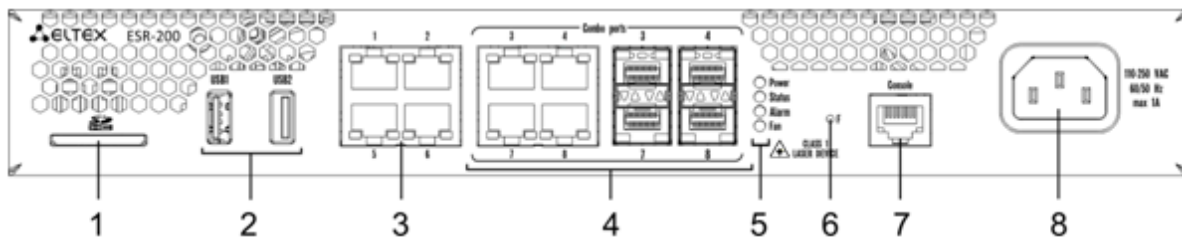
Рисунок 32 – Передняя панель ESR-200
