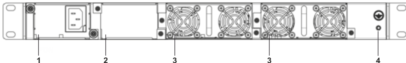
Рисунок 29 – Задняя панель ESR-1200, ESR-1000
