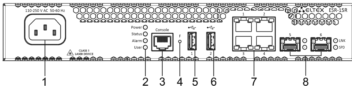
Рисунок 54 – Передняя панель ESR-15R
