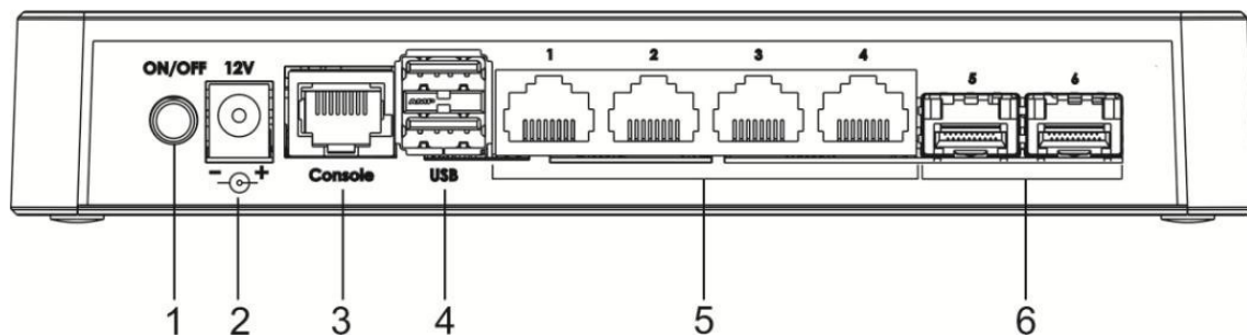
Рисунок 68 – Задняя панель ESR-10
