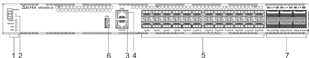
Рисунок 28 – Передняя панель MES5400-24
