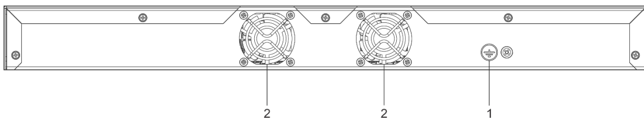
Рисунок 39 – Задняя панель MES2300-24P
