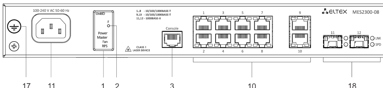
Рисунок 1 – Передняя панель MES2300-08
