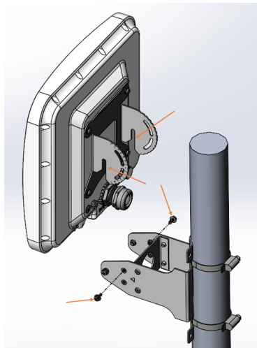
Рисунок 9 — Установка устройства на зафиксированный кронштейн
