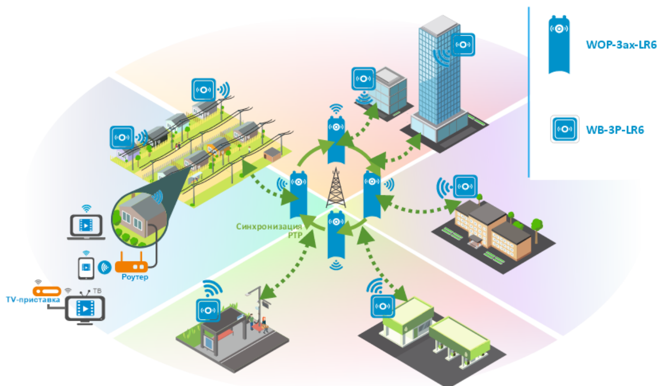
Рисунок 23 — Схема применения WB-3P-LR6
