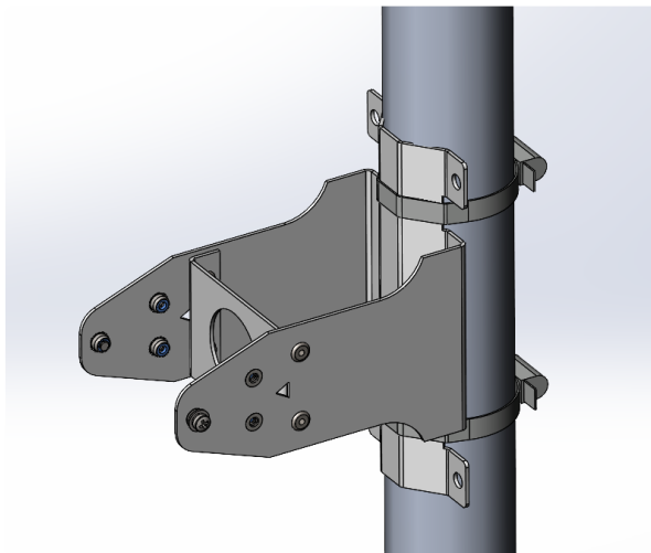
Рисунок 7 (а) — Вертикальная установка
