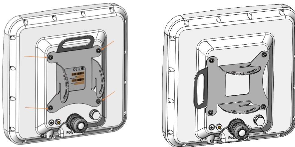
Рисунок 5 — Крепление подвижной части кронштейна к устройству
