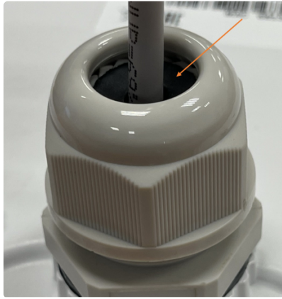
Рисунок 20 — Затягивание гайки кабельного ввода
