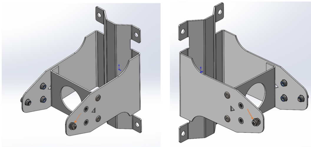
Рисунок 6 — Установка винтов в неподвижную часть кронштейна
