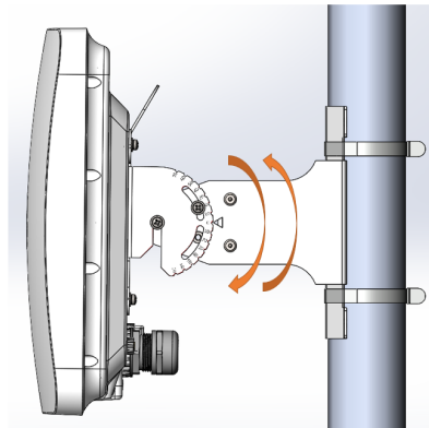
Рисунок 22 — Настройка необходимого угла наклона
