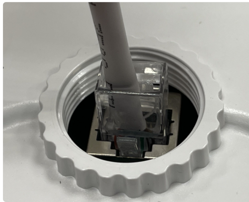
Рисунок 18 — Подключение Ethernet-кабеля к PoE-порту
