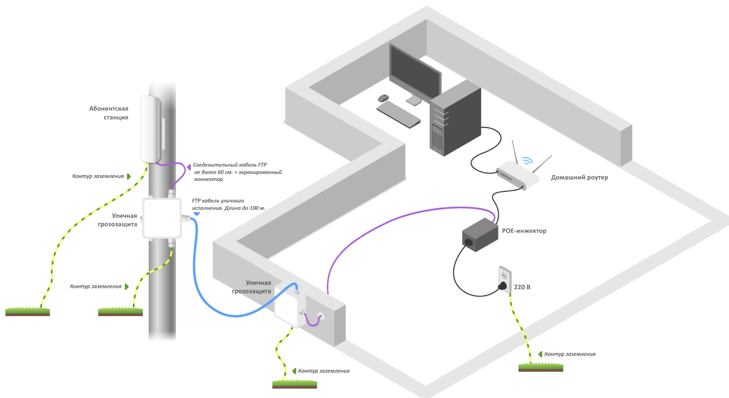
Схема подключения абонентской станции для обеспечения грозозащиты
