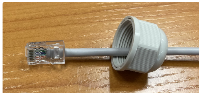
Рисунок 13 — Установка гайки кабельного ввода на кабеле
