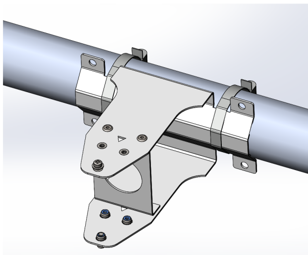
Рисунок 7 (б) — Горизонтальная установка
