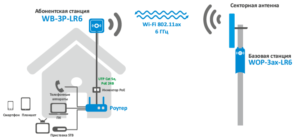
Рисунок 1 — Функциональная схема использования WB-3P-LR6
