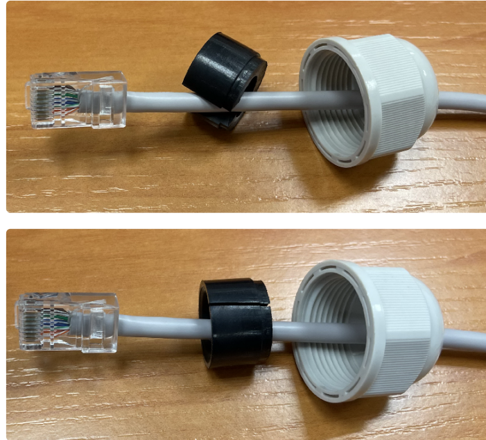
Рисунок 14 — Установка резиновой втулки на кабеле
