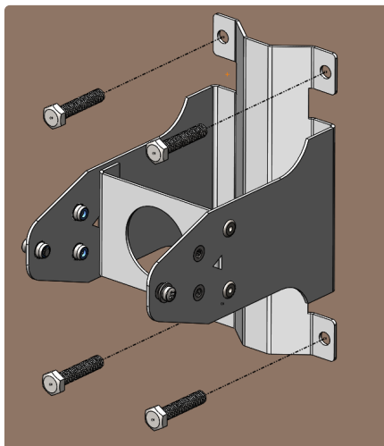
Рисунок 8 (а) — Вертикальная установка
