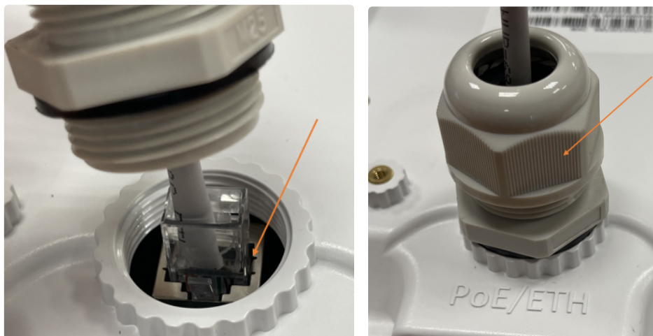
Рисунок 19 — Установка кабельного ввода в корпус устройства
