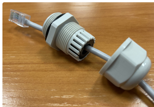
Рисунок 16 — Установка резиновой втулки в корпус кабельного ввода
