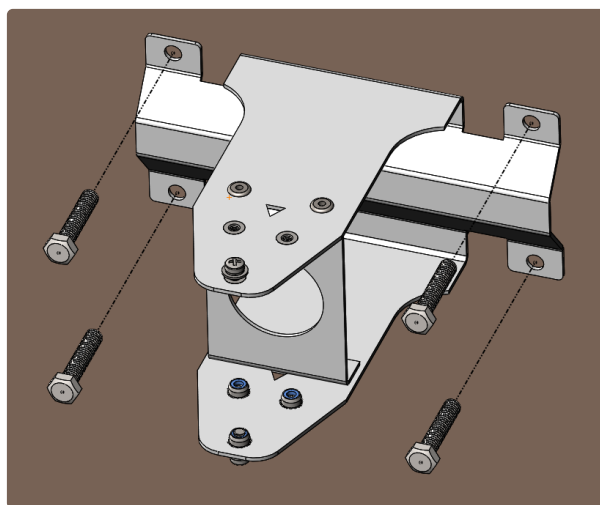
Рисунок 8 (б) — Горизонтальная установка
