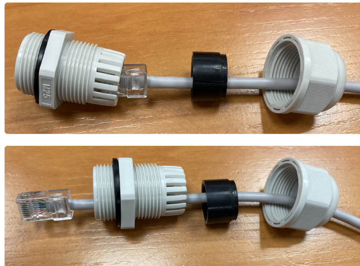
Рисунок 15 — Установка корпуса кабельного ввода на кабеле
