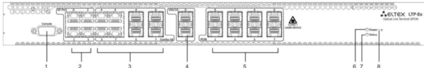
Рисунок 1 – Передняя панель LTP rev.B
