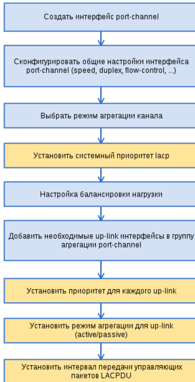
Рисунок 28 — Последовательность настройки LAG и LACP
