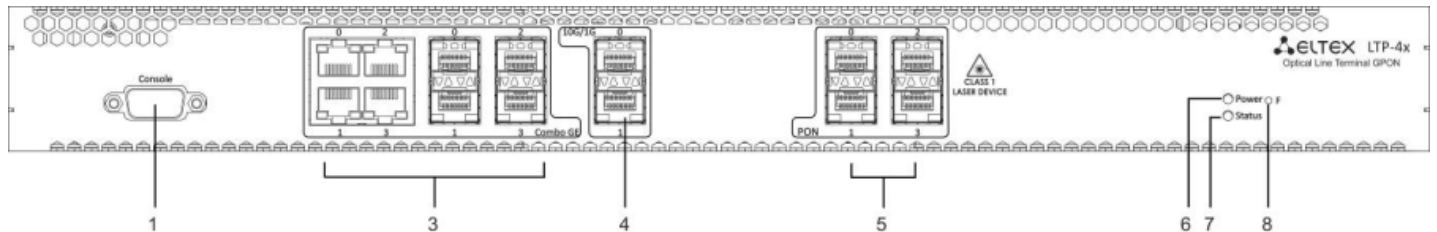
Рисунок 1 – Передняя панель терминала LTP-4X rev.B
