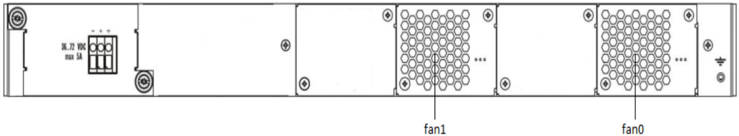
Рисунок 5 — Задняя панель станционного терминала LTP-4X/8X (DC)
