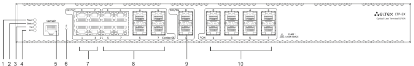
Рисунок 4 – Передняя панель терминала LTP-8X rev.C/rev.D
