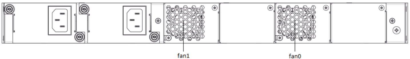
Рисунок 7 — Задняя панель станционных терминалов LTP-4X/8X rev.C, LTP-4X/8X rev.D с двумя блоками питания
