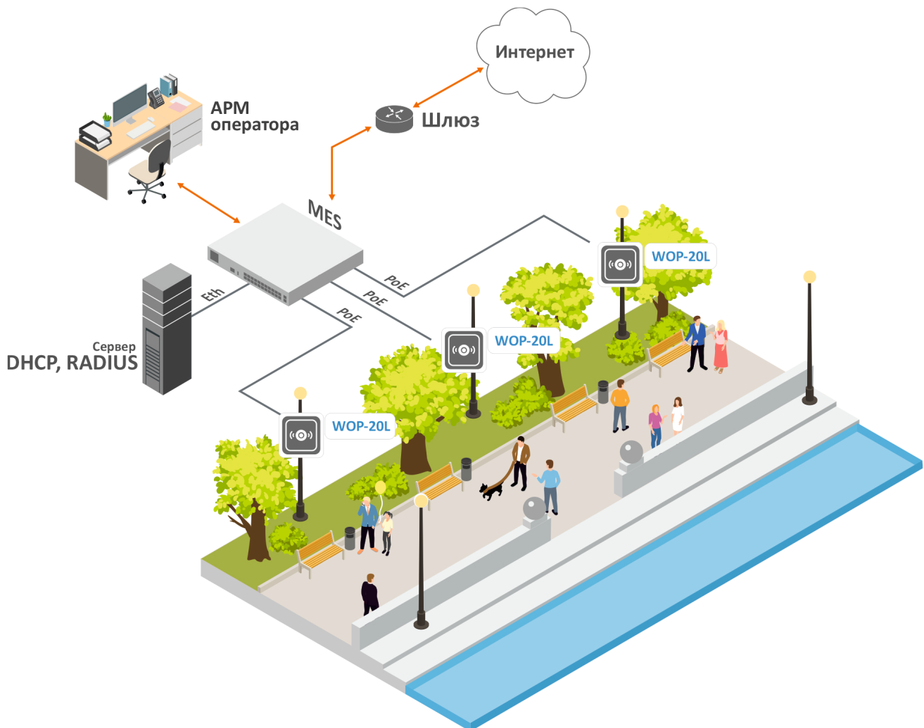
Рисунок 1 — Функциональная схема использования WOP-20L
