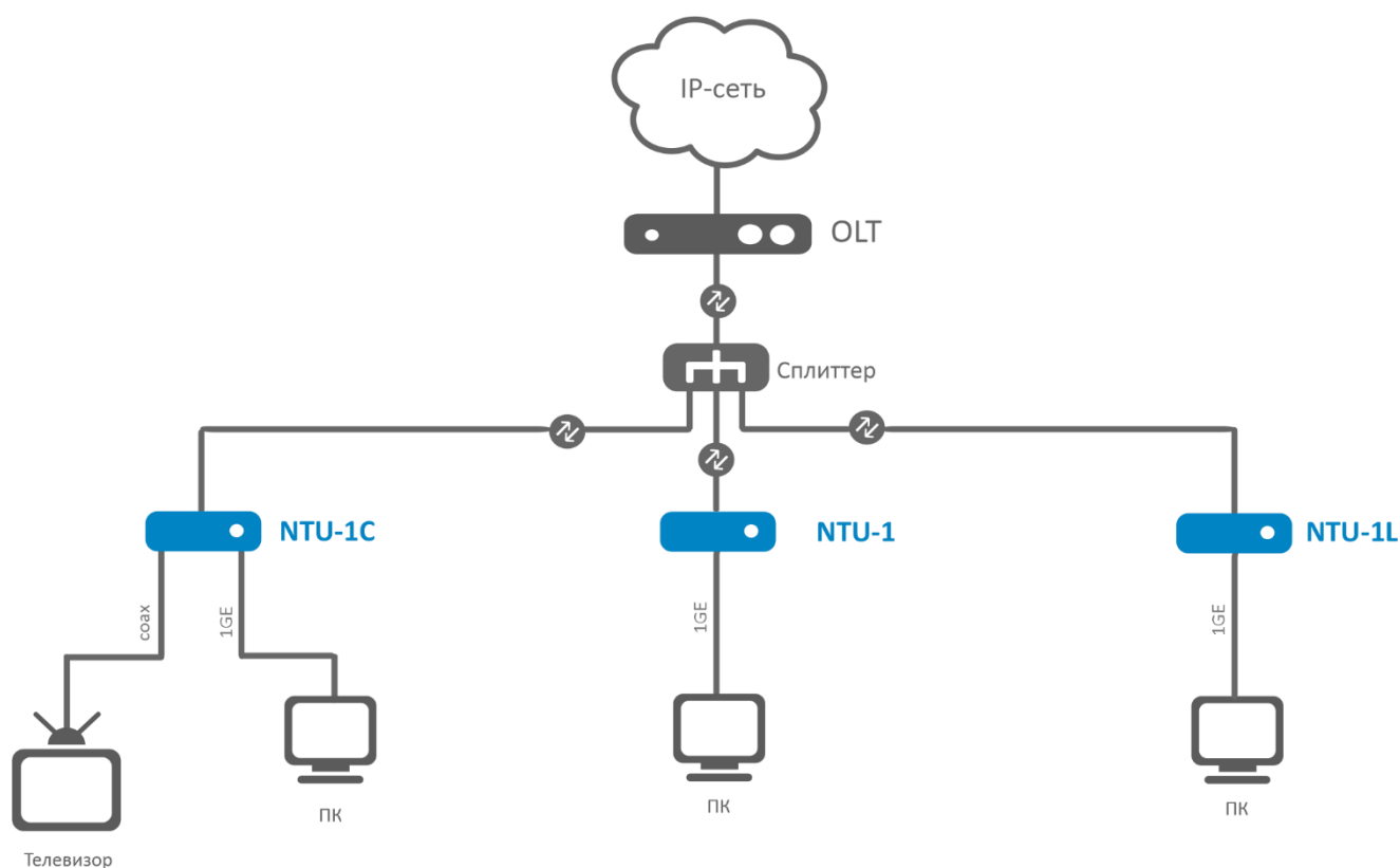
Рисунок 1 — Схема применения NTU-1, NTU-1C, NTU-1L
