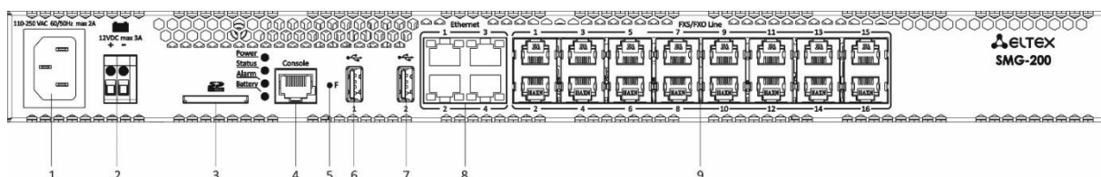
Рисунок 6 — Внешний вид передней панели SMG-200
