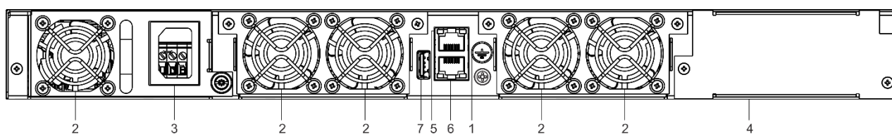
Рисунок 56 – Задняя панель MES5300-48, MES5305-48, MES5310-48
