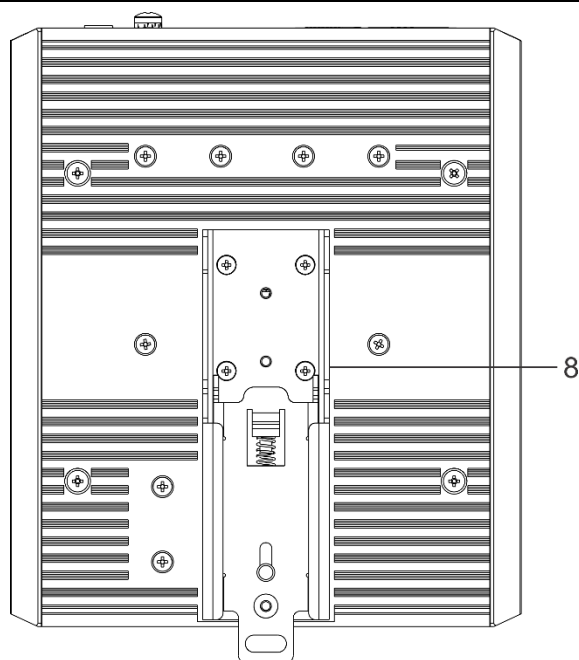
Рисунок 53 – Задняя панель MES3500I-8P8F
