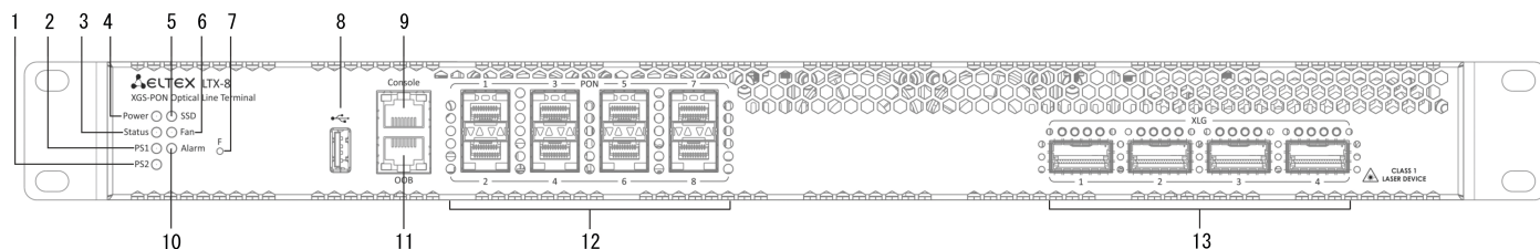
Рисунок 9 – Передняя панель терминала LTX-8
