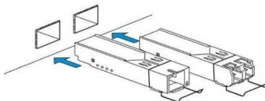
Рисунок 43 – Установка SFP-трансиверов
