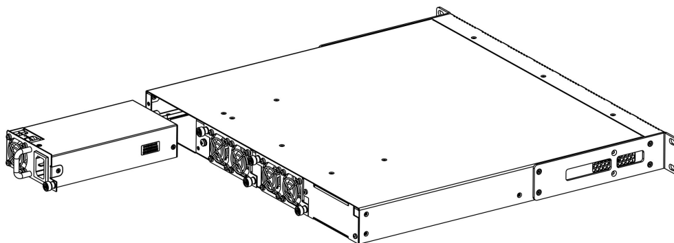
Рисунок 19 – Установка модуля питания LTX-8(16), LTX-8(16) rev.B
