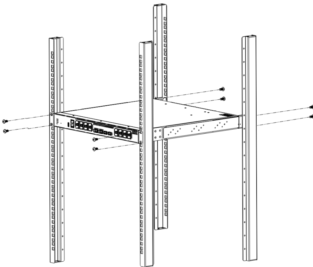
Рисунок 26 – Установка LTX-8(16)C в стойку
