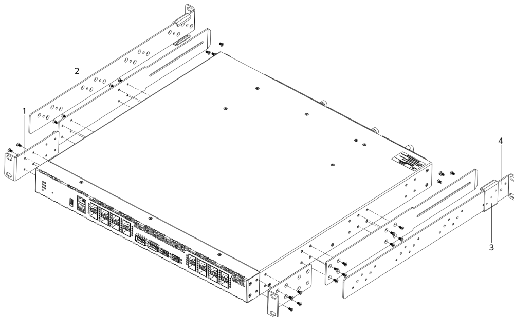
Рисунок 25 – Крепление кронштейнов LTX-8(16)C
