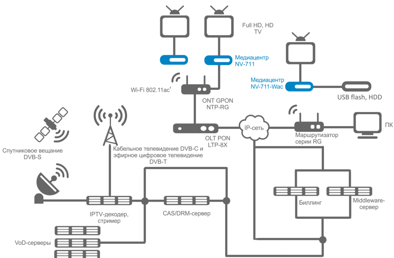
Рисунок 1 – Схема применения
