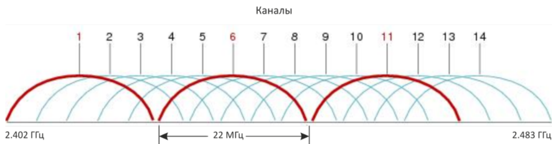
Рисунок 5 — Общая диаграмма перекрытия частотных каналов в 2.4 ГГц
