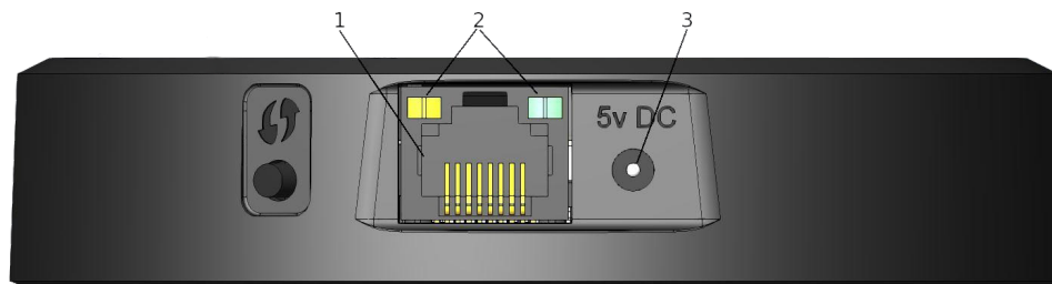
Рисунок 3 — Внешний вид задней панели WEP-1L
