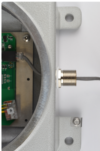
Рисунок 15 — Подключение Ethernet-кабеля
