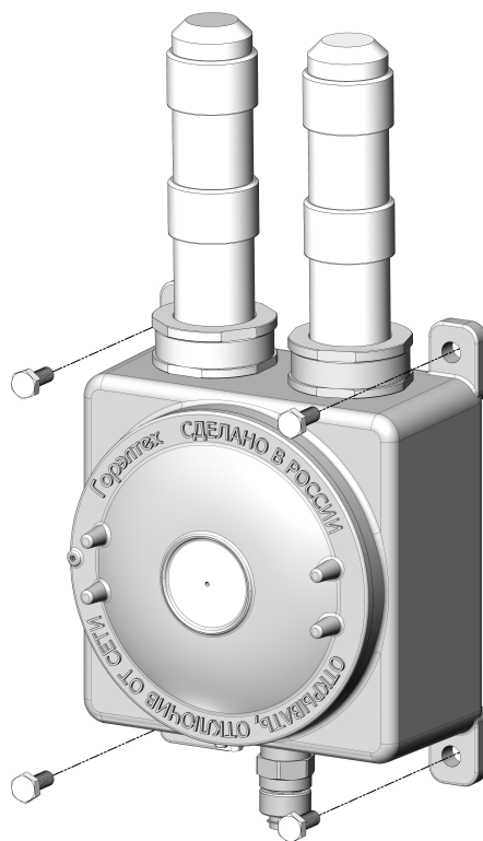
Рисунок 8 — Крепление устройства при помощи болтового соединения
