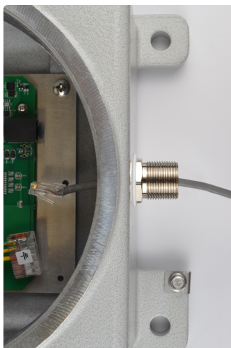
Рисунок 14 — Кабель с коннектором RJ-45
