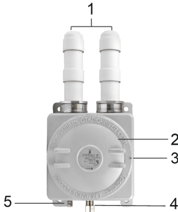
Рисунок 2 — Внешний вид основной панели WOP-3L-EX
