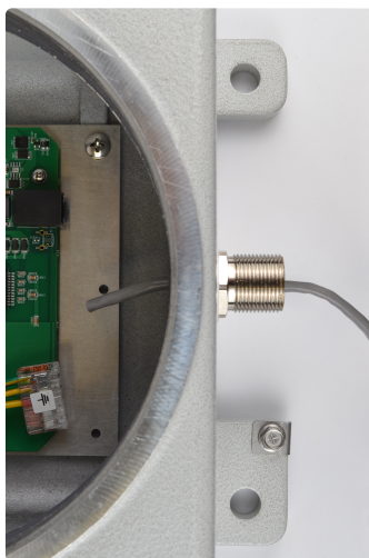
Рисунок 13 — Протяжка кабеля через кабельный ввод
