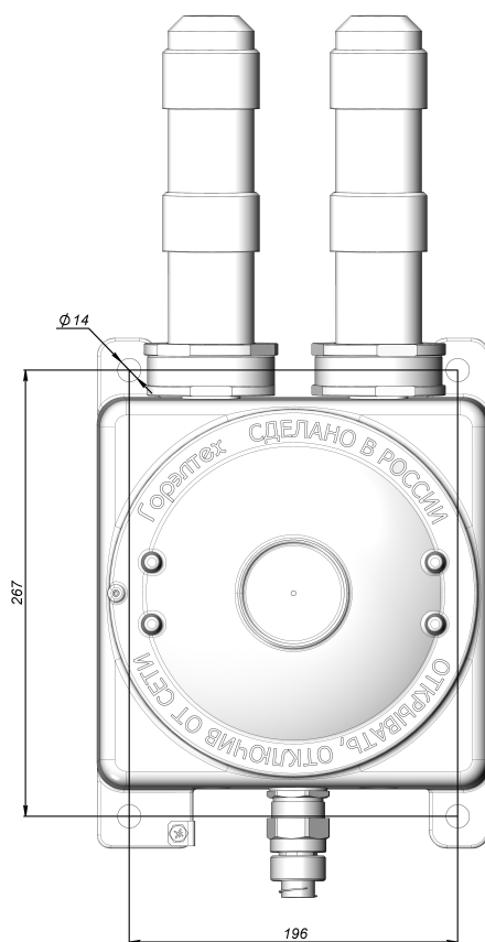
Рисунок 7 — Присоединительные размеры
