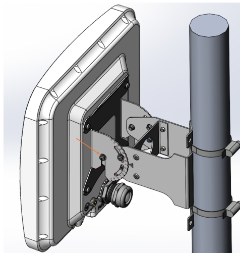
Рисунок 11 — Фиксация винтов
