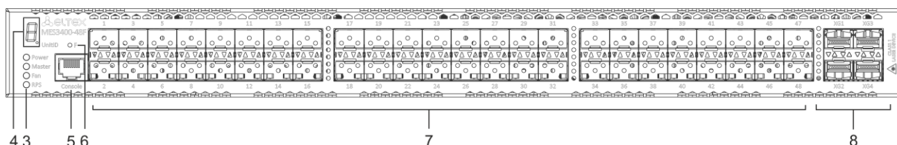
Рисунок 31 – Передняя панель MES3400-48F
