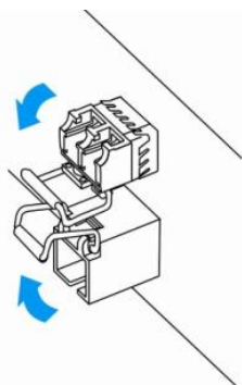
Рисунок 62 – Открытие защелки SFP-трансиверов
