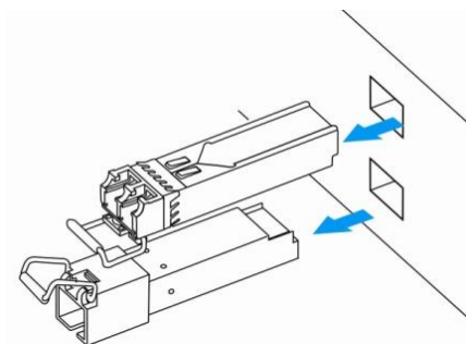
Рисунок 63 – Извлечение SFP-трансиверов
