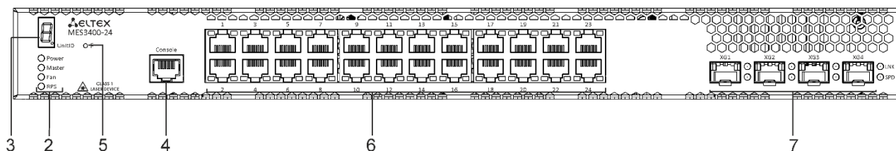
Рисунок 26 – Передняя панель MES3400-24
