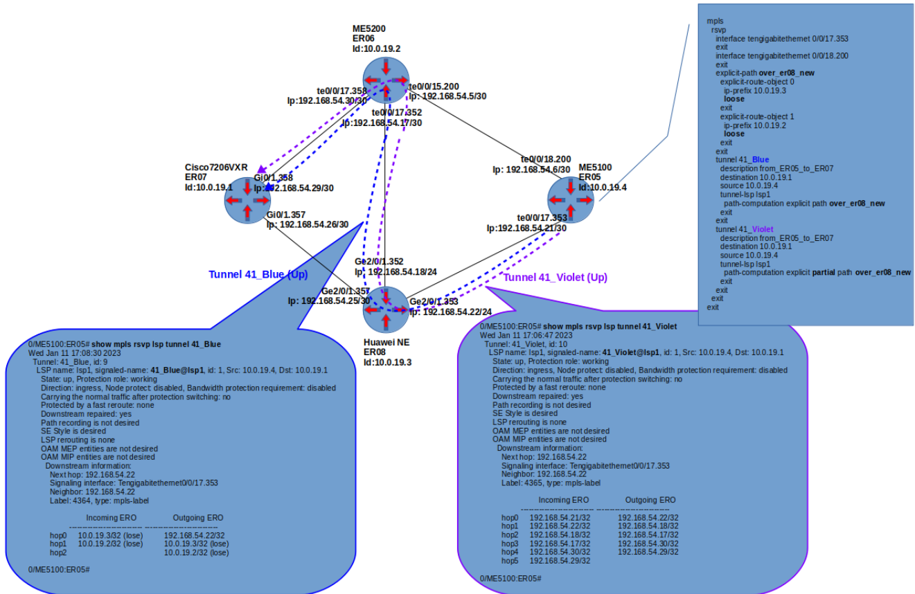
Figure 3. Конфигурация TE-туннелей с explicit path и опциям loose и partial.
