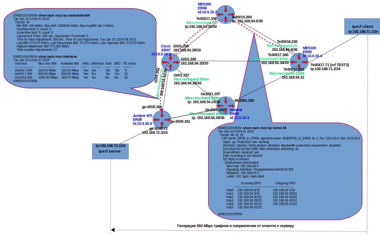
Figure 11. Как построится RSVP LSP 46@ER05_to_ER09 при генерации трафика 550 Mbps.
