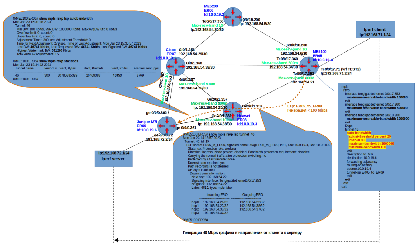
Figure 9. Начальное положение RSVP LSP 46@ER05_to_ER09 при генерации трафика до 100 Mbps.
