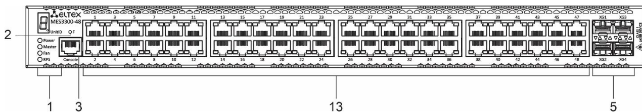
Рисунок 16 – Передняя панель MES3300-48
