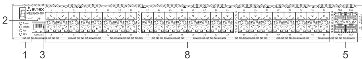
Рисунок 17 – Передняя панель MES3300-48F
