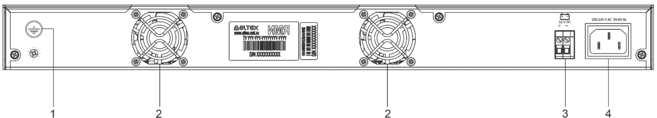
Рисунок 36 – Задняя панель MES2300B-48
