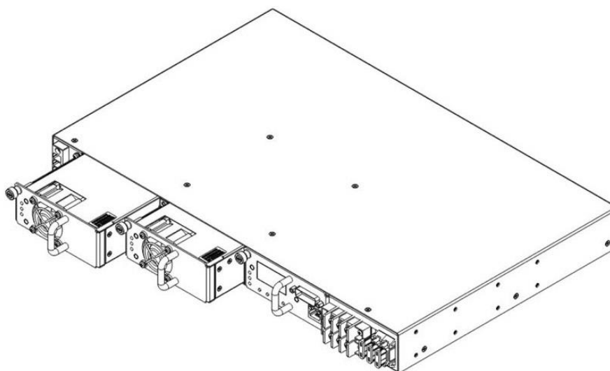
Рисунок 10 – Установка модулей питания
