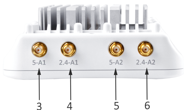
Рисунок 4 – Внешний вид верхней панели WOP-20L
