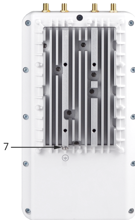
Рисунок 5 – Внешний вид задней панели WOP-20L
